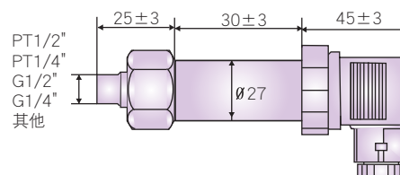
尺寸圖 單位: mm
