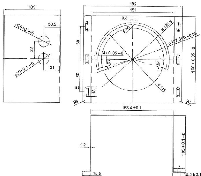
型號(TYPE):D4E6A
