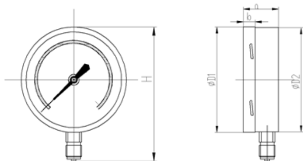
Ø6" 型式 B : 直立式 IP65
