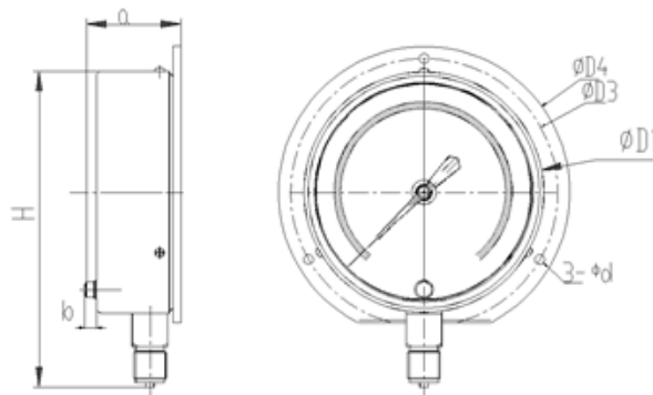
Ø6" 型式 W : 壁掛式(3 螺絲孔背緣) IP54
