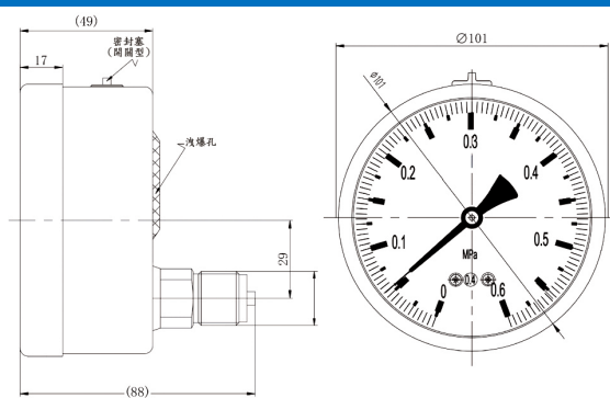
Ø4" 型式 DE : 背接式 偏心牙 IP65
