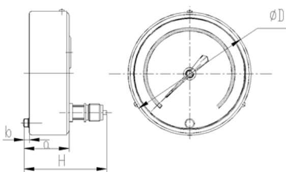
Ø6" 型式 DE : 背接式 偏心牙 IP54
