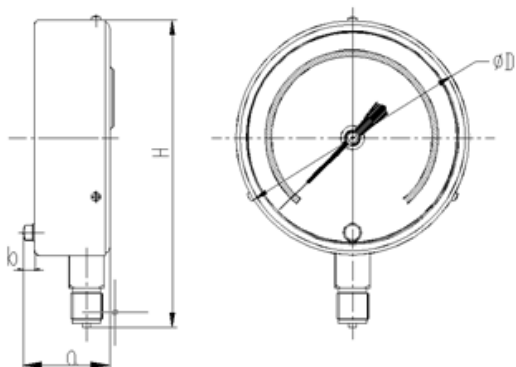
Ø6" 型式 B : 直立式 IP54
