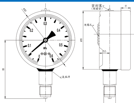
Ø4" 型式 B : 直立式 IP65
