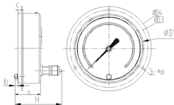
Ø6" 型式 PE : 埋入附三孔邊 背接偏心牙 IP54
