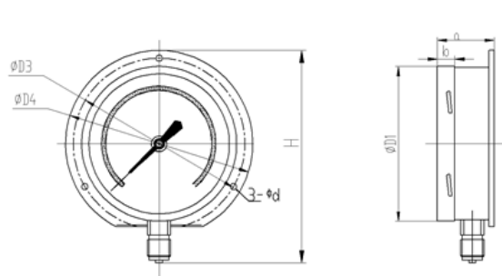
Ø6" 型式 W : 壁掛式(3 螺絲孔背緣) IP65
